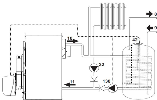
Отопление + БГВ с помпа
