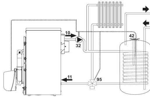
Отопление + БГВ с 3-пътен вентил
