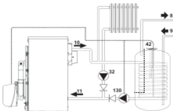
Отопление + БГВ с помпа
