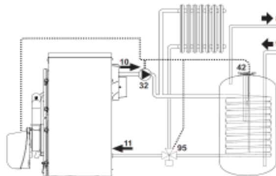
Отопление + БГВ с 3-пътен вентил
